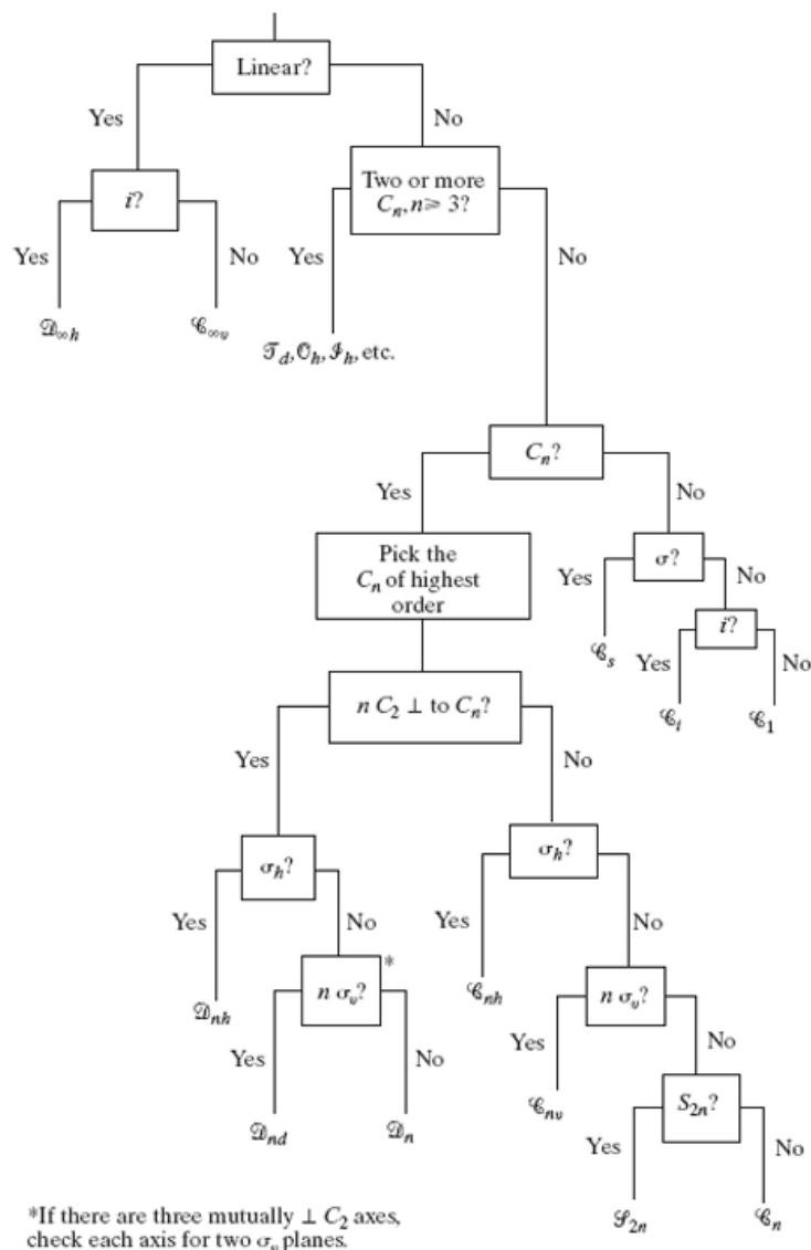
图 12.15: 确定分子所属点群步骤示意图。
